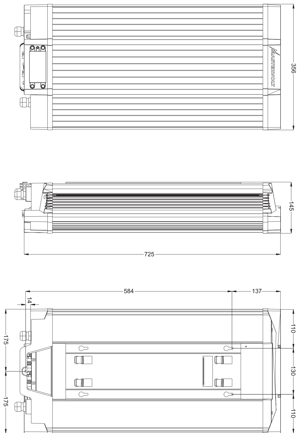
Afbeelding 29: Afmetingen van de Sunmaster XS6500
