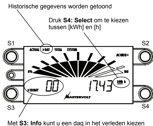
Afbeelding 25: Historische gegevens
