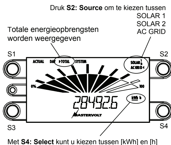
Afbeelding 26: Totale energieopbrengst
