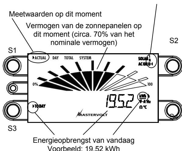
Afbeelding 23: beginscherm (getoonde meetwaarden kunnen afwijken)
