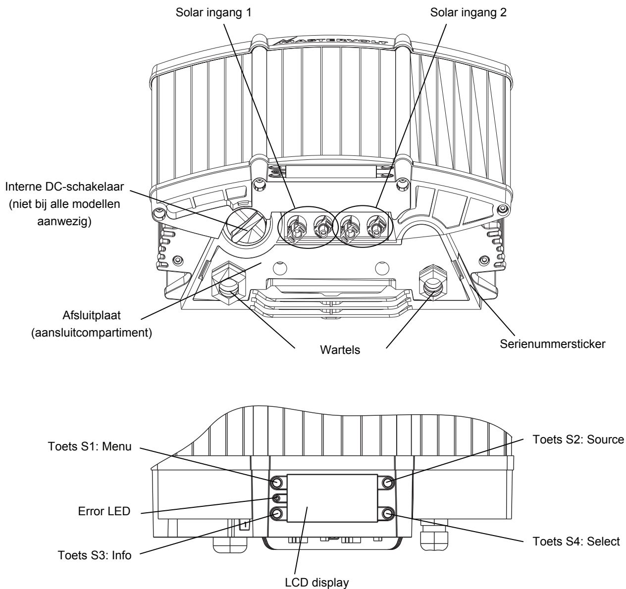
Afbeelding 1: overzicht van de Mastervolt Sunmaster XS6500
